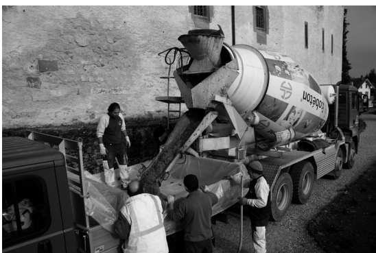
Livraison du béton pour l'escalier de secours: du gros camion au petit camion
